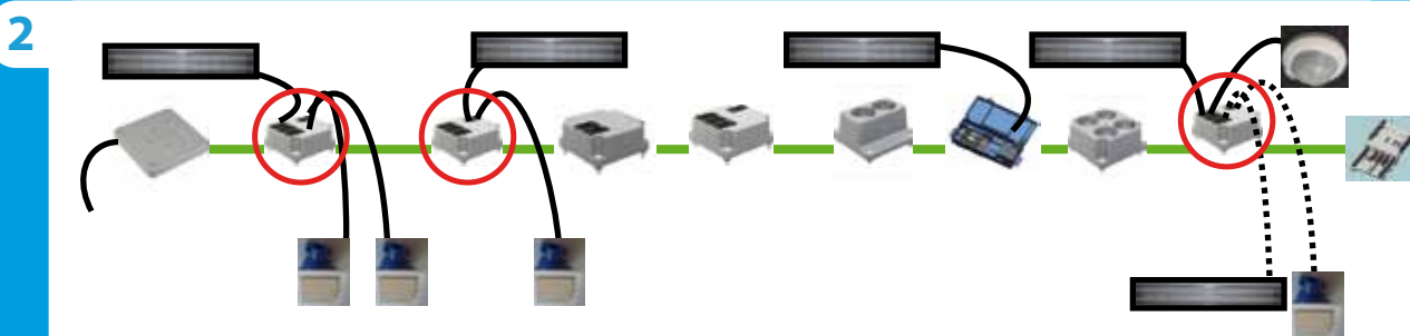
3G installatie met schakelunits
