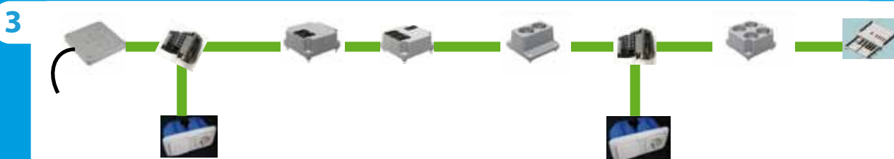
5G Kabel installatie wisselschakelaars
